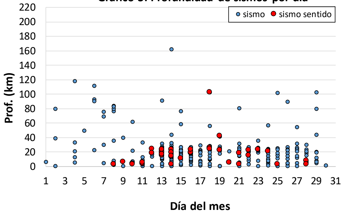
Gráfico 3: Profundidad de sismos por día
