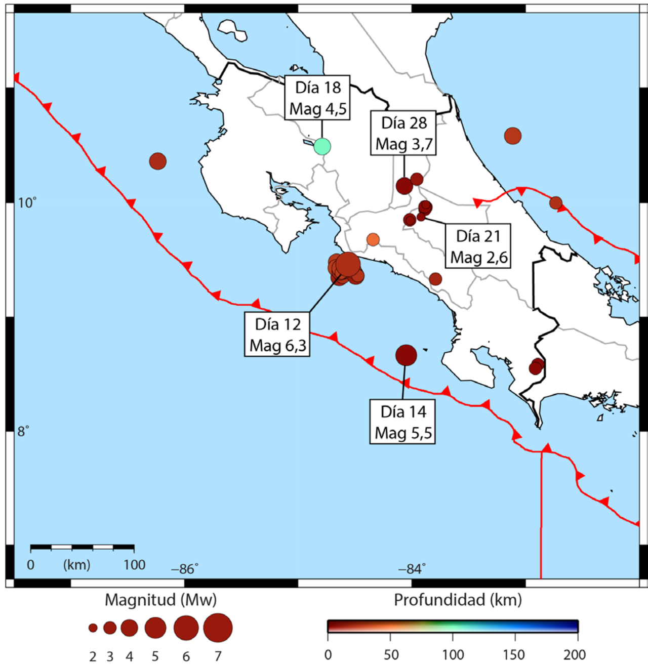
Figura 2: Sismos sentidos durante noviembre del 2017
