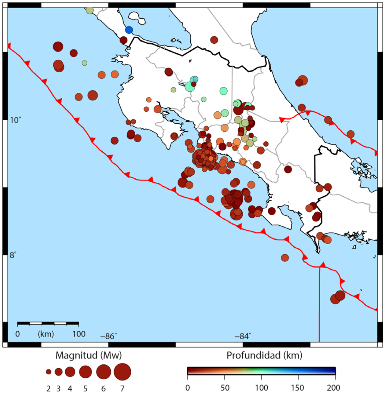
Figura 1: Sismos localizados por la RSN durante noviembre del 2017
