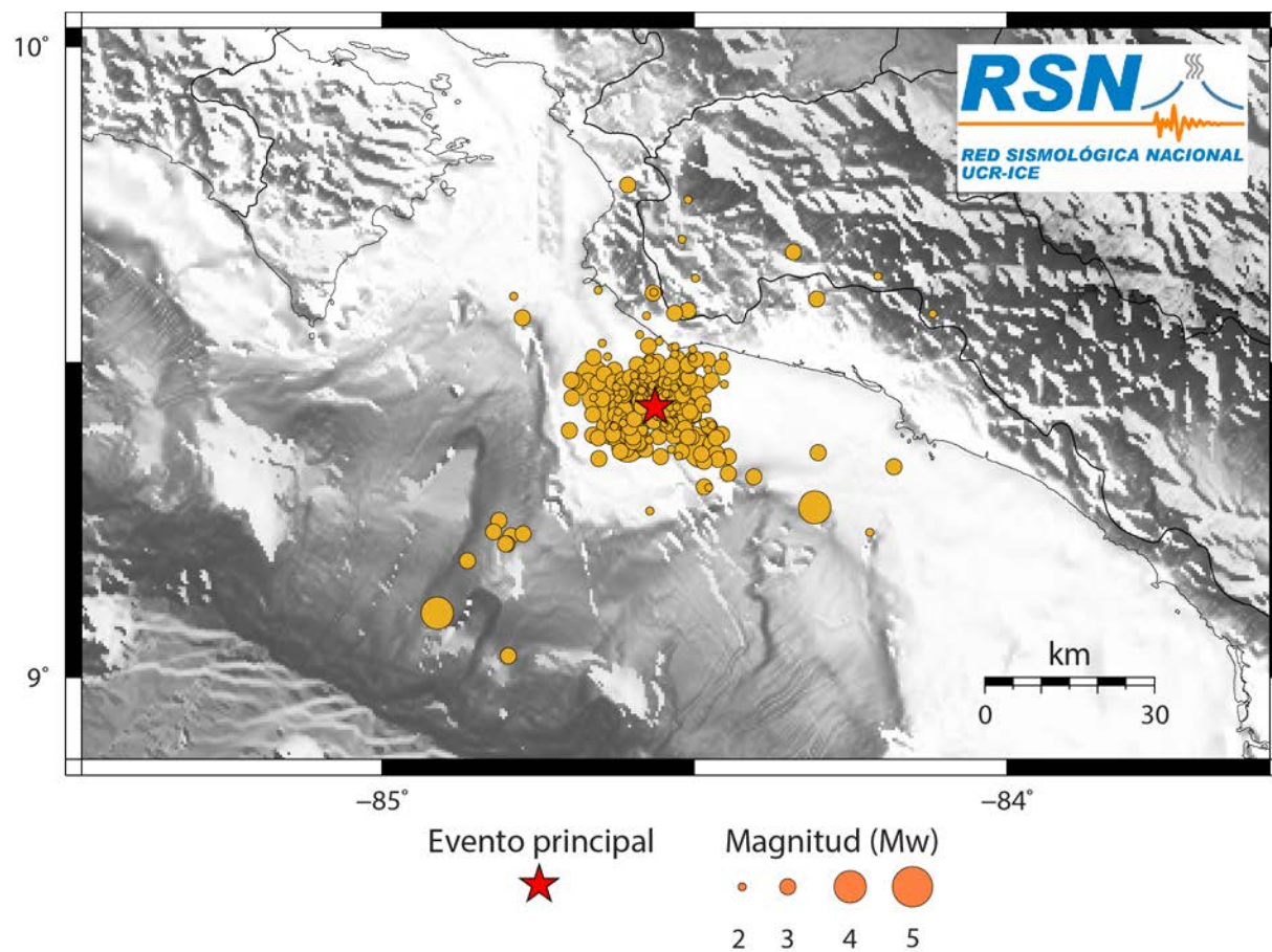
Figura 4: Secuencia sísmica del sismo de Jacó (Mw 6,3) del 12 de noviembre, y 280 réplicas localizadas con precisión hasta la fecha.
