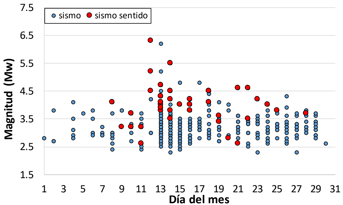
Gráfico 4: Magnitud de sismos por día
