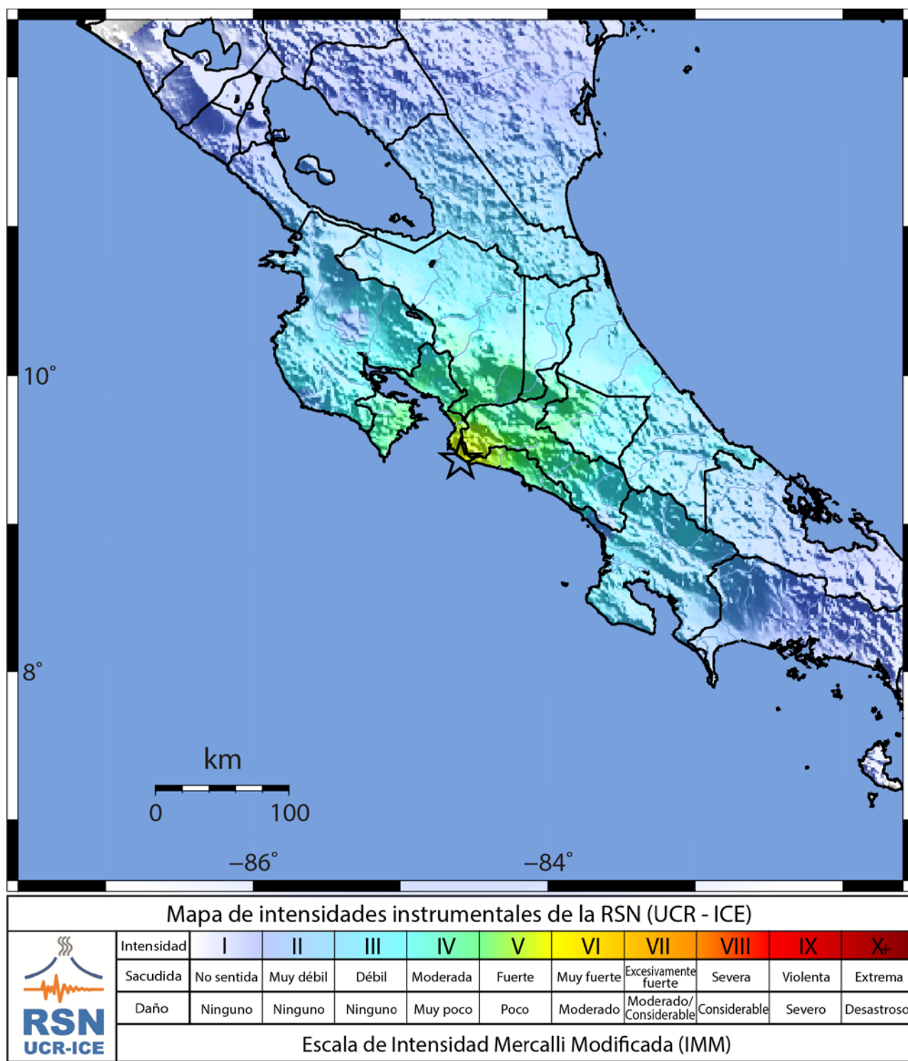
Figura 3: Intensidades máximas registradas por la red de instrumentos de la RSN durante noviembre del 2017
